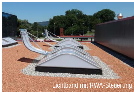
Vier Lichtkuppeln eines RWA-Systems
